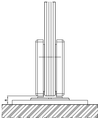
Spodní řez stěnou
