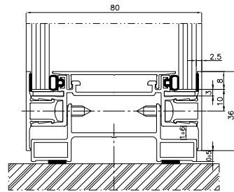
Spodní řez stěnou
