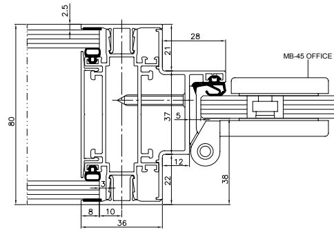
Vodorovný řez stěnou s dveřmi MB-45 OFFICE
