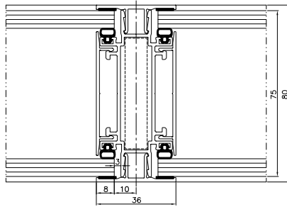
Svislý řez stěnou 80 mm
