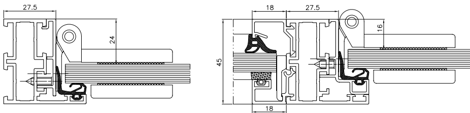
Řez sloupků dveří
