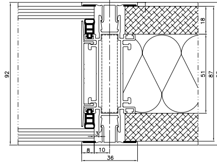
Svislý řez stěnou 92 mm
